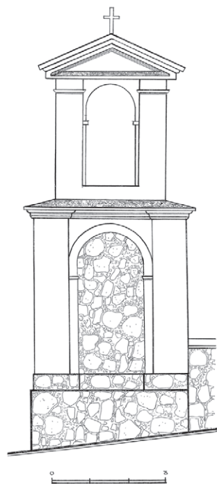
4 pav. Aleksandravėlės varpinės galinis fasadas. Atliko A. Rupeika
