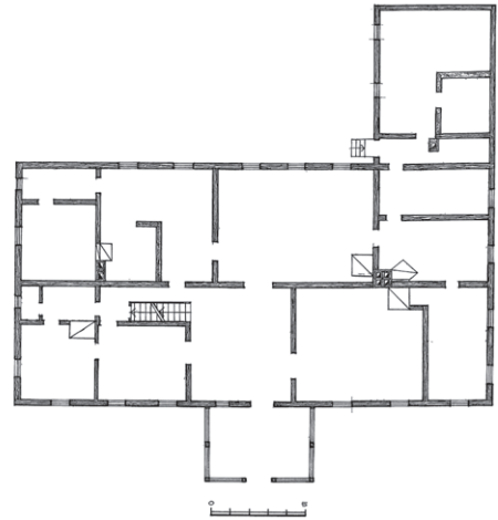
11 pav. Obelių klebonijos planas. Sudarė A. Rupeika
