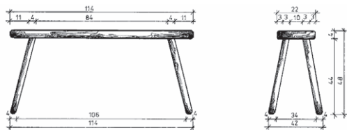
6 pav. Suolelis. Gamintas apie 1890 m. Dačiūnų k. (Obelių sen.). Piešė Kristina Navickaitė. 1980 m.
