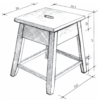
9 pav. Taburetė. XX a. 3-iasis dešimtmetis. Dačiūnų k. (Obelių sen.). Piešė Irida Drejerytė. 1980 m.
