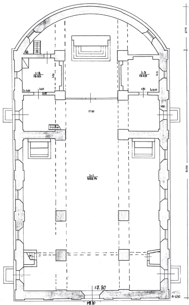
Kriaunų Dievo Apoaidos bažnyčios planas
