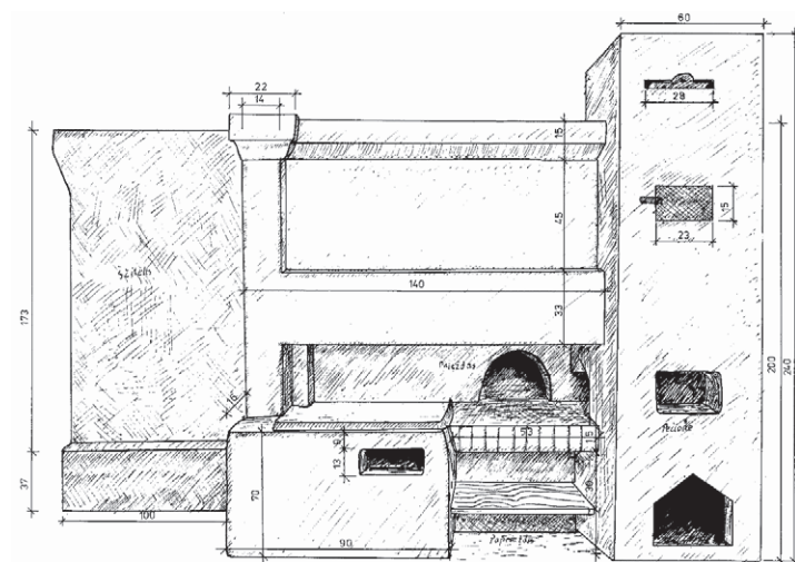
2 pav. Krosnis, statyta XX a. 2-ame dešimtmetyje Kavolių k. (Panemunėlio sen.). Piešė Gintaras Zalagėnas. 1979 m.
