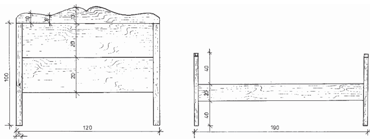
10 pav. Lova. XIX a. pab. Bučelių k. (Obelių sen.). Piešė D. Černogolovainaitė ir D. Petukauskaitė. 1980 m.
