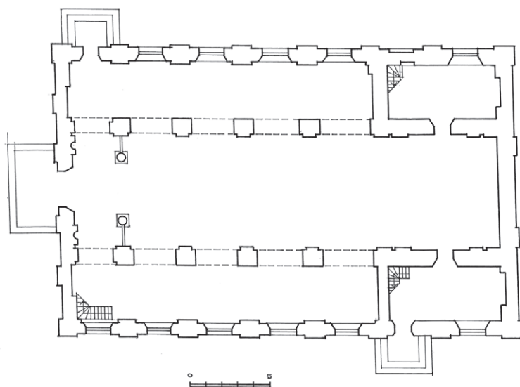
2 pav. Aleksandravėlės bažnyčios planas. Sudarė A. Rupeika
