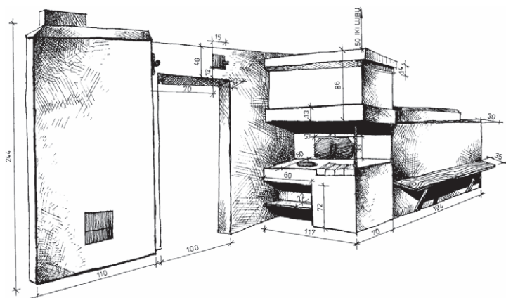
1 pav. Krosnis, statyta 1887 m. Arlaučiznos k. (Kriaunų sen.). Piešė Robertas Čerškus. 1980 m.
