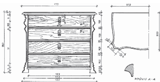
17 pav. Komoda. XX a. pr. Rudžionių k. (Obelių sen.). Piešė D. Šarakauskas. 1980 m.
