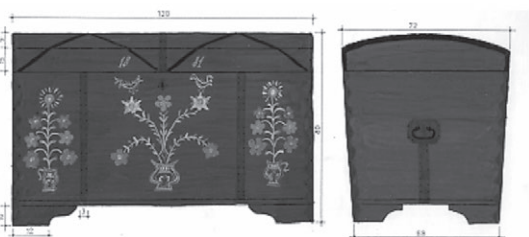
15 pav. Skrynja dėžiniu antvožu (kupas). XIX a. Degenių k. (Kazliškio sen.). Piešė Virginija Kalinauskaitė. 1979 m.
