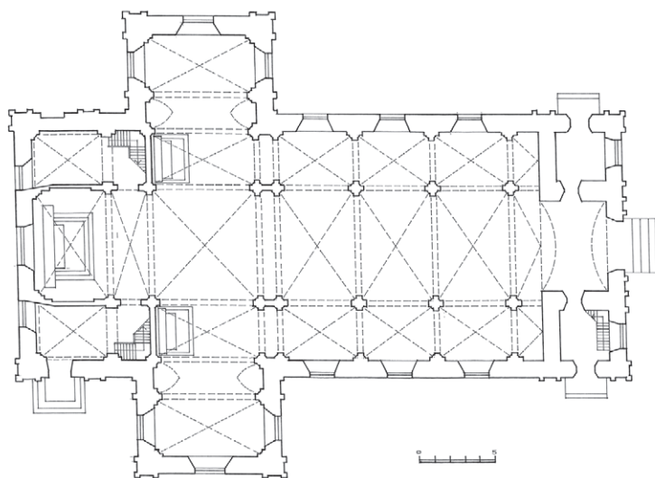
10 pav. Obelių bažnyčios planas. Sudarė A. Rupeika
