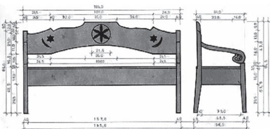
7 pav. Suolas su atlošu. XIX a. pab. Navikų k. (Obelių sen.). Piešė Dalius Šarakauskas. 1980 m.
