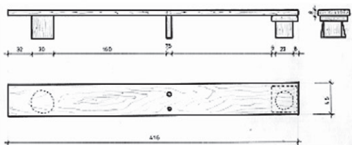
5 pav. Gryčios suolas. XIX a. pab. Meldeikiškio k. (Panemunėlio sen.). Piešė G. Zalagėnas. 1979 m.
