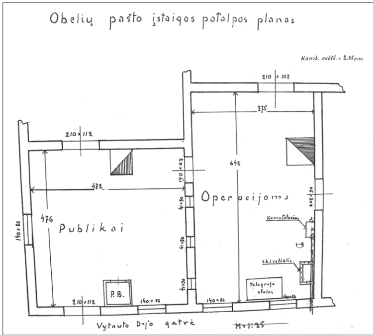
Obelių pašto 1929–1933 m. patalpų planas. LCVA, f. 1016, ap. 2, b. 114
