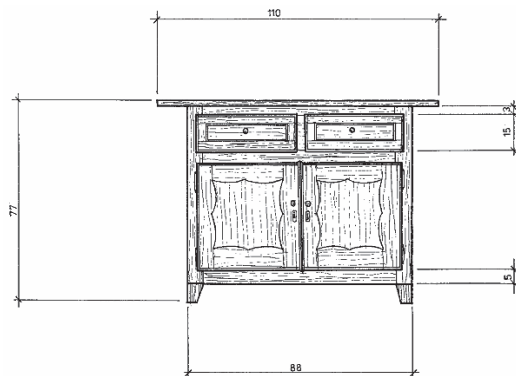
13 pav. Spintelė. XX a. pr. Lukiškių k. (Panemunėlio sen.). Piešė Mindaugas Čepas. 1979 m.
