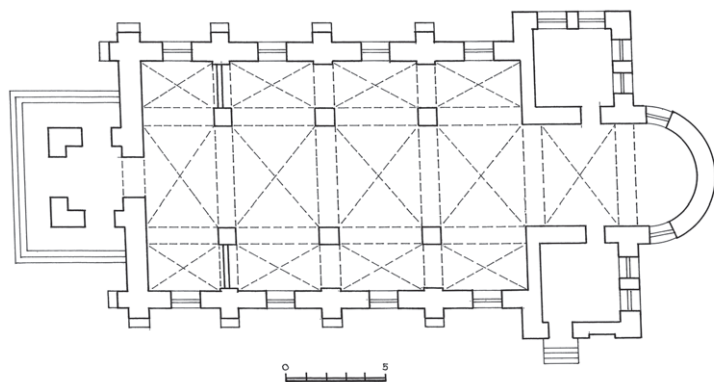
8 pav. Lukštų bažnyčios planas. Sudarė A. Rupeika
