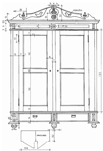
18 pav. Rūbų spinta. XX a. pr. Skemų k. (Rokiškio sen.). Piešė D. Černogolovinė ir D. Petukauskaitė. 1980 m.
