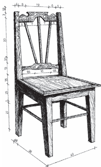
8 pav. Kėdė. XX a. pr. Arlaučiznos k. (Kriaunų sen.). Piešė N. Šalčiūtė. 1980 m.
