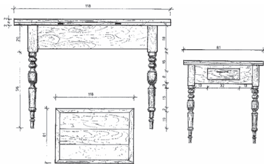
4 pav. Seklyčios stalo. Gamintas apie 1930 m. Palūgės k. (Obelių sen.). Piešė D. Černogolovainaitė ir Daiva Petukauskaitė. 1980 m.
